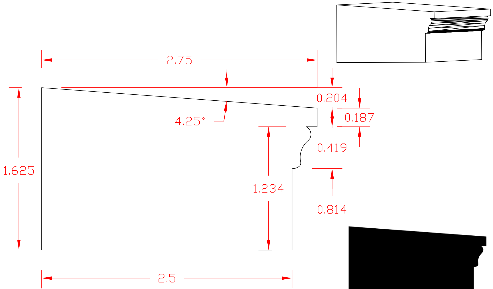
2-3/4" DOOR HEADER CAP ATW-3062
